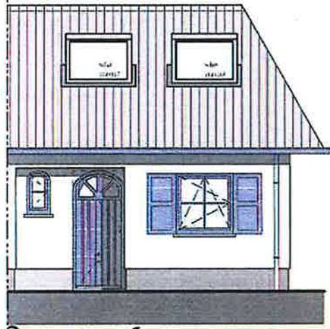
Voorgevel
